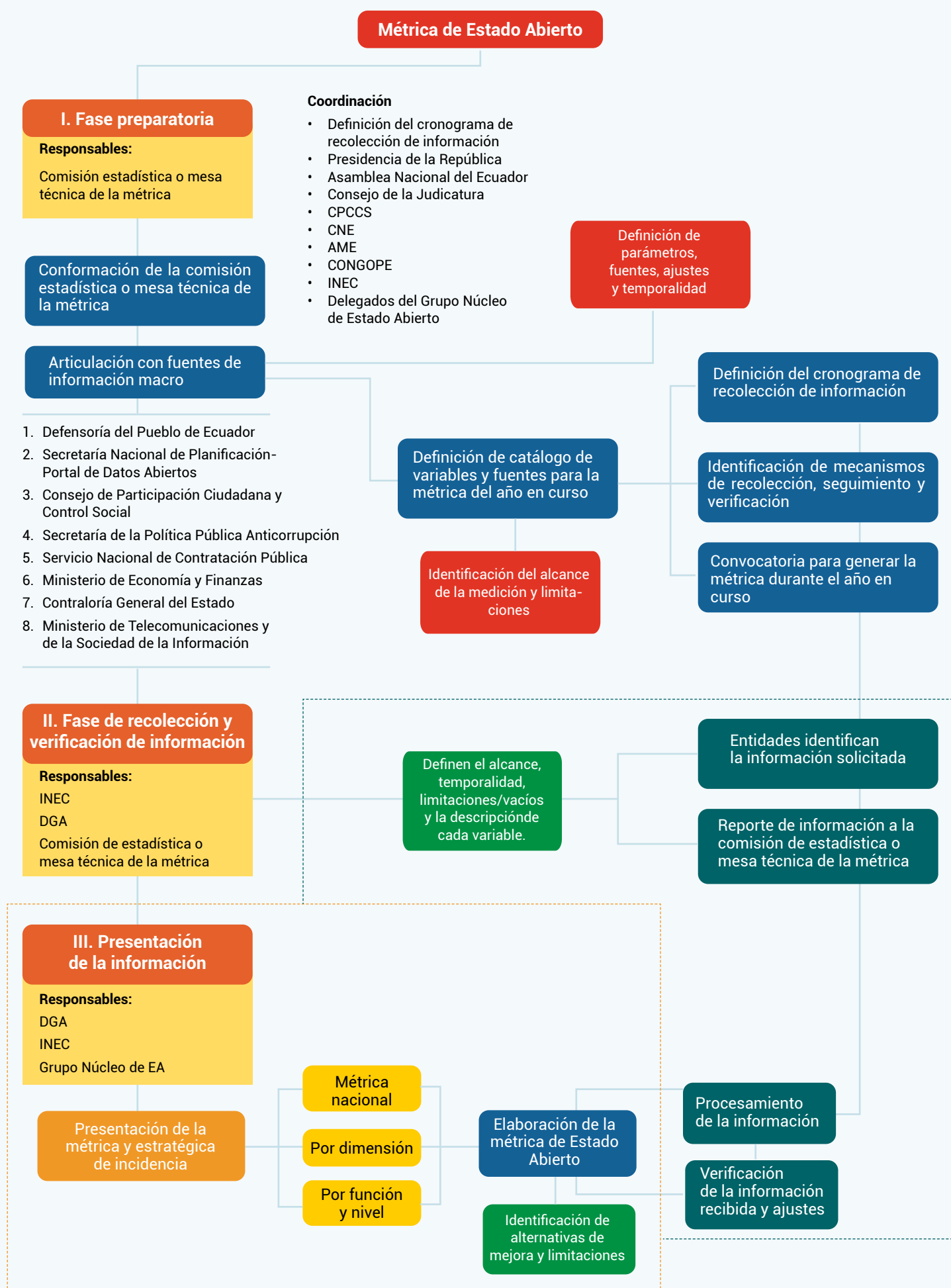
Gráfico 1. Flujograma propuesto para construir la métrica
